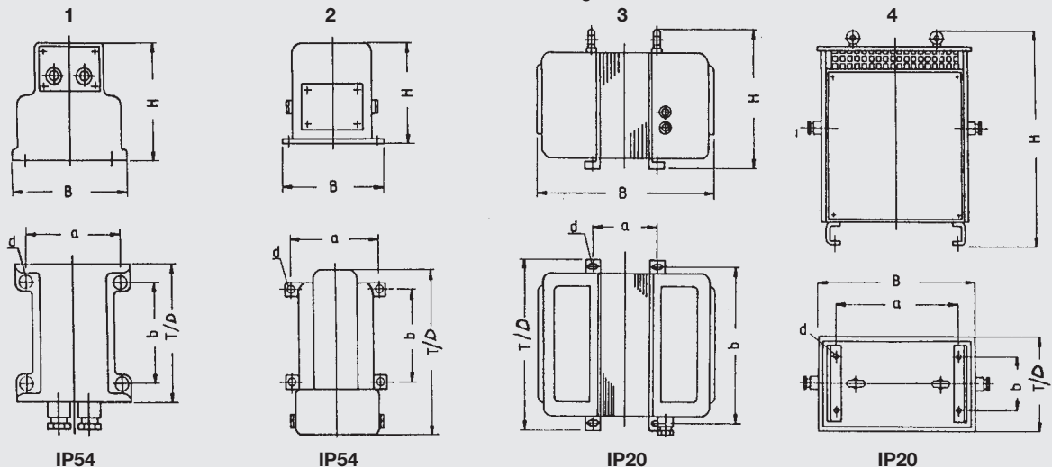
Maßbild/Drawing
